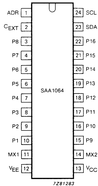
Fig.2 Pinning diagram.
