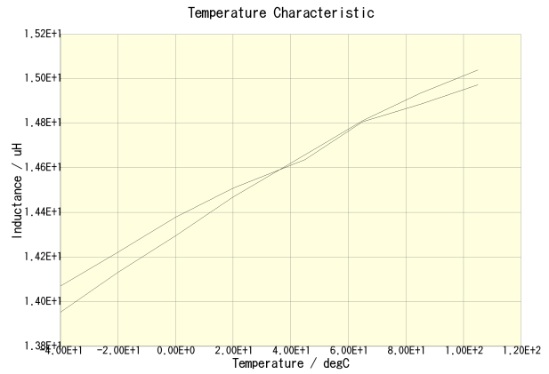
SLF10145T-150M2R2-PF(DC = 0A) SLF10145T-150M2R2-PF(DC = 1.1A)
